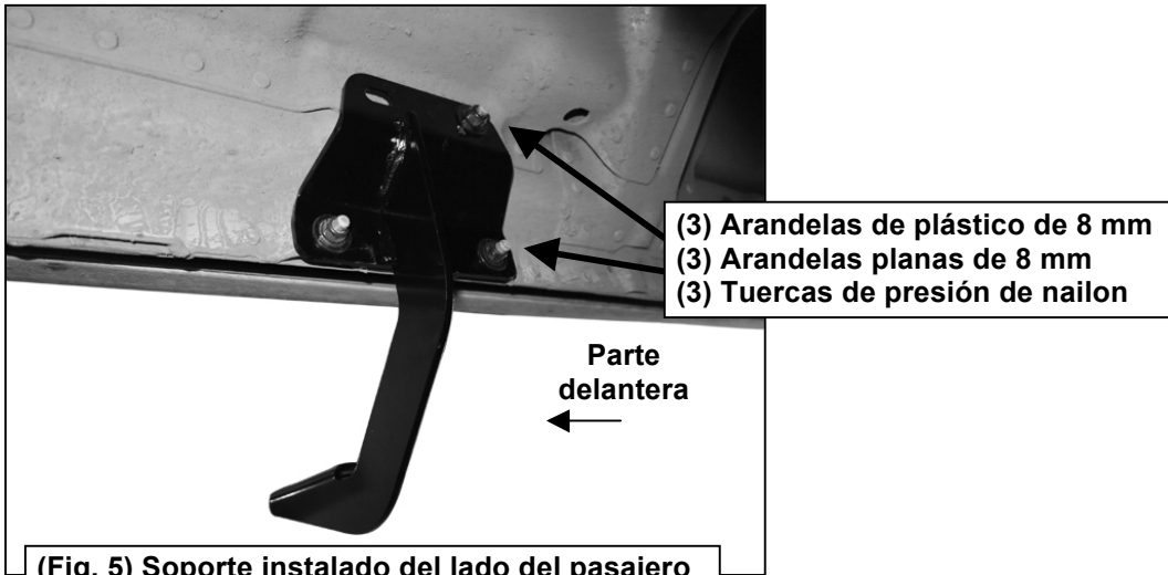
(Fig. 5) Soporte instalado del lado del pasajero delantero
