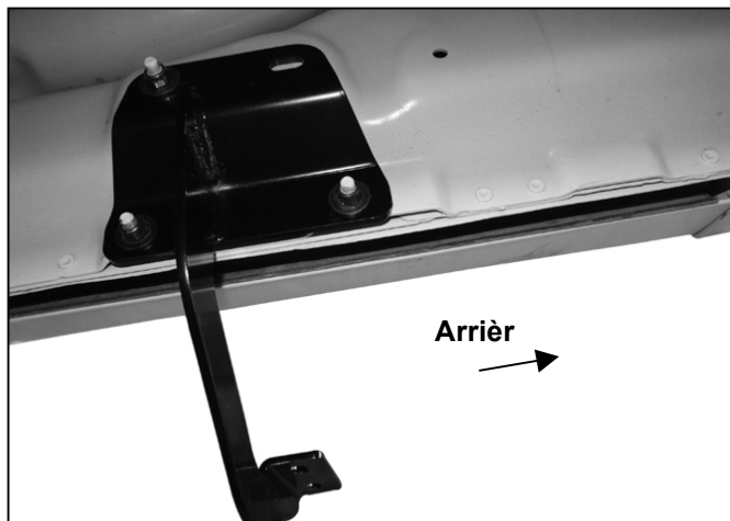
(Fig. 6) Support arrière du côté passager installé
