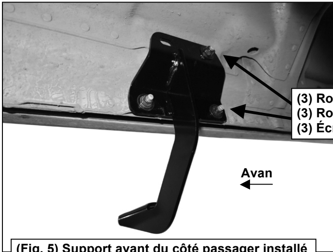
(Fig. 5) Support avant du côté passager installé
