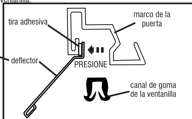
Vista del corte transversal del deflector ubicado en su lugar
